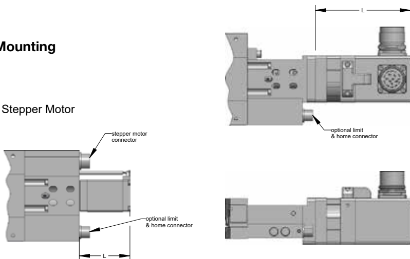
Servo Motor
