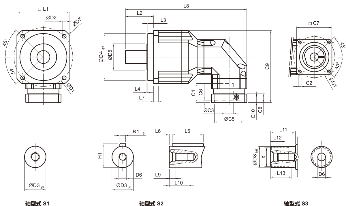
轴型式 S1
