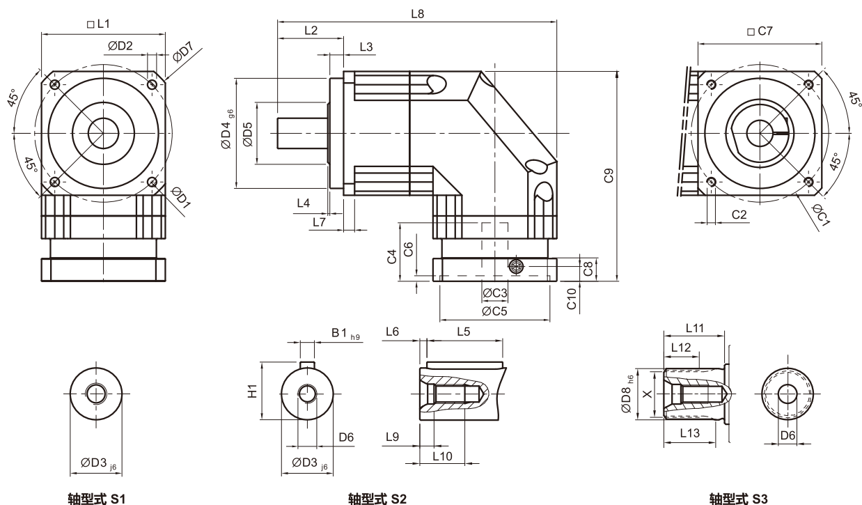
轴型式 S1
