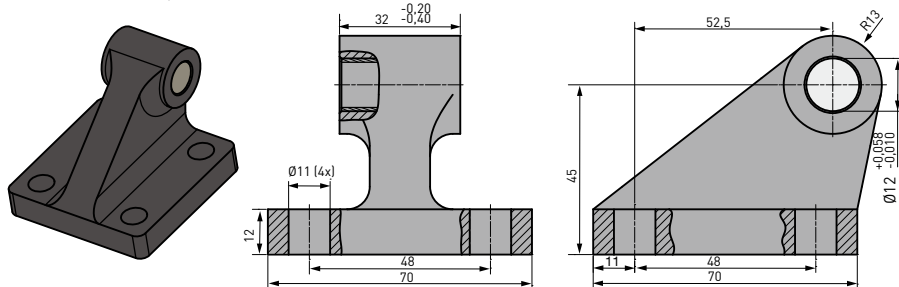
ETH080的轴承座, 部件编号. 0132.039
